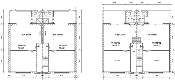
Begane grond bestaande/nieuwe toestand ongewijzigd (schaal 1:100)
