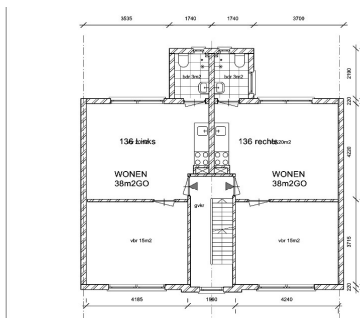
2/3e verdieping bestaande toestand (schaal 1:100)
