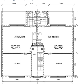
1e verdieping bestaande toestand (schaal 1:100)
