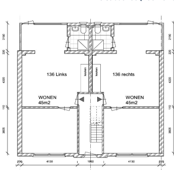
Begane grond bestaande/nieuwe toestand ongewijzigd (schaal 1:100)
